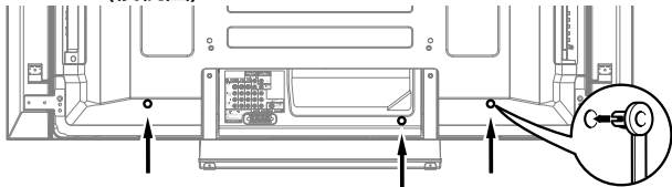
PDP-508XG (後視圖)
